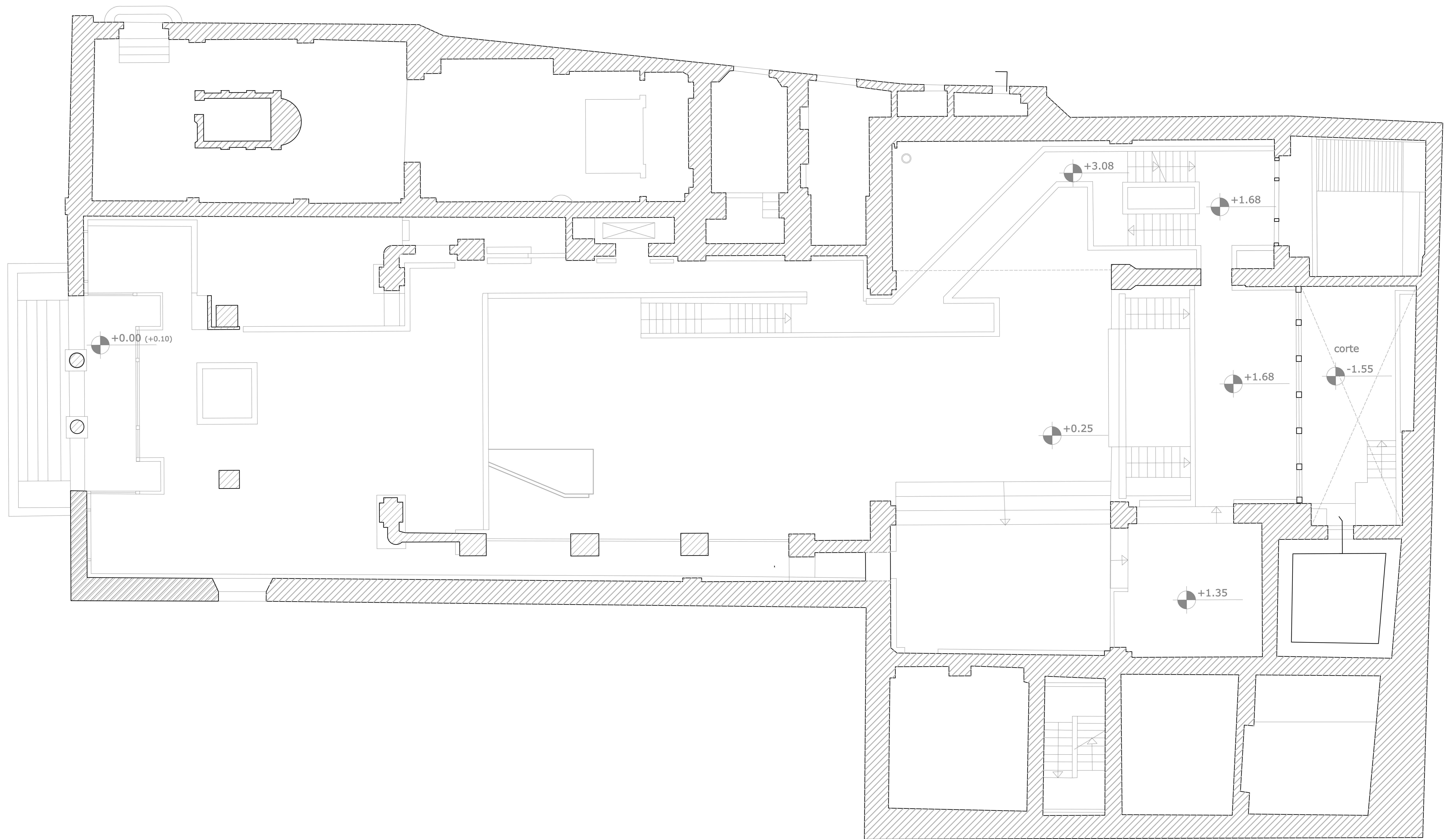
Pianta Piano Ammezzato +3.08
